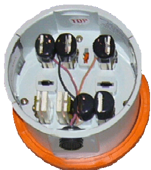
Meter Socket Adapter 12S or 15S
